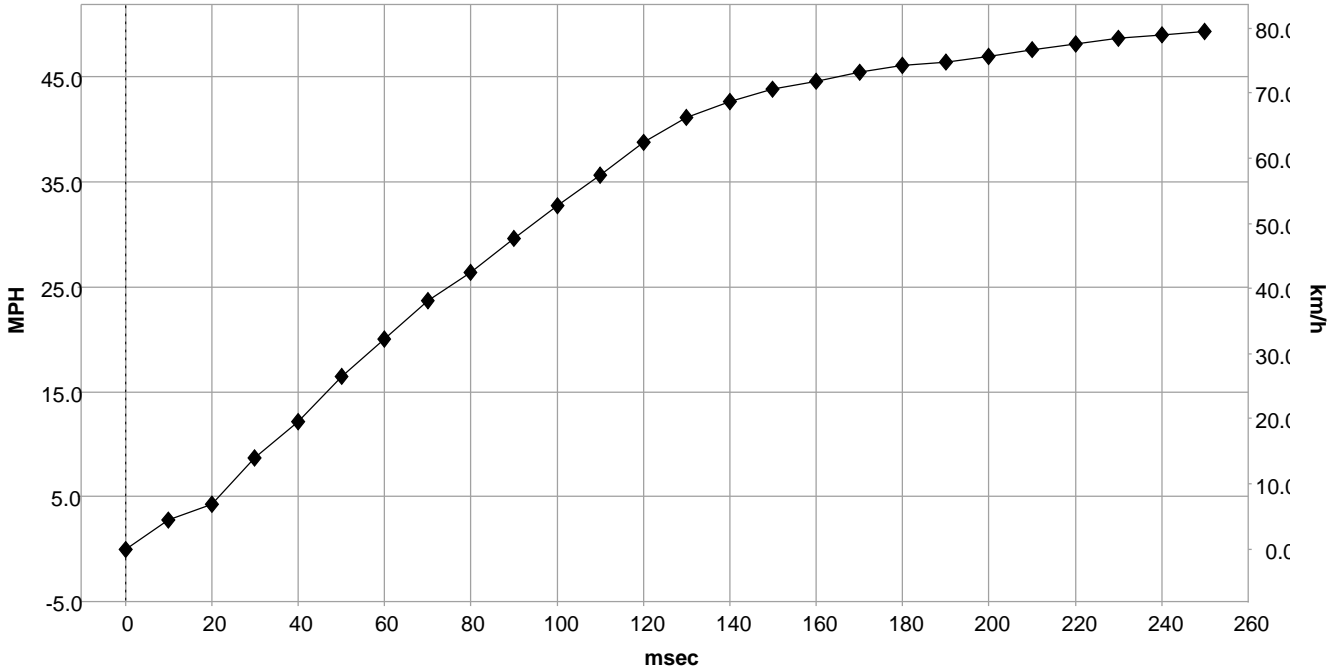
Longitudinal Delta-V
