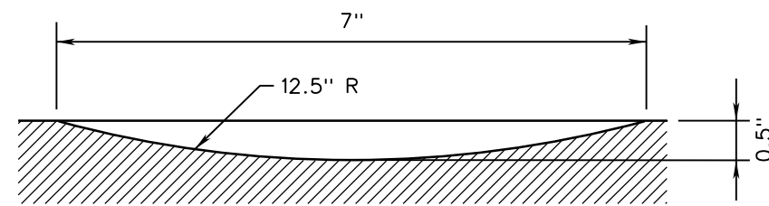
RUMBLE GROOVE SECTION B-B
