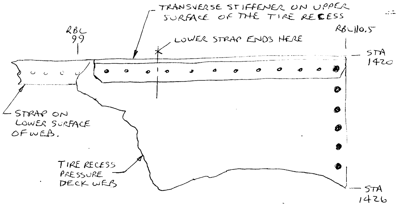
VIEW A-A
