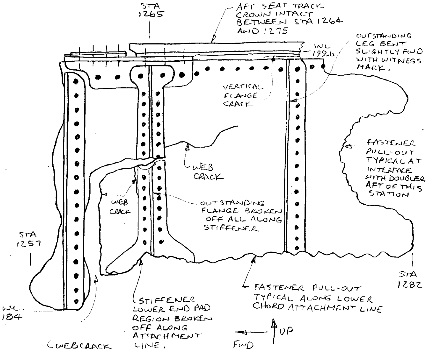
VIEW A-A
