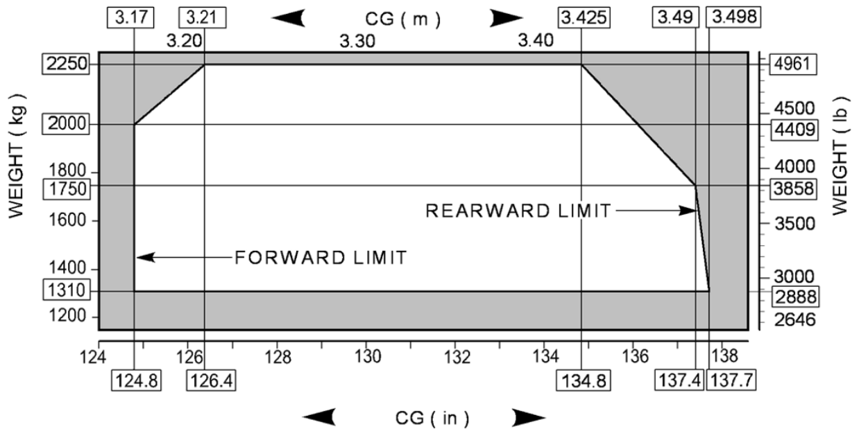
CG (in) Longitudinal: AS350 B3 ARRIEL 2D:
