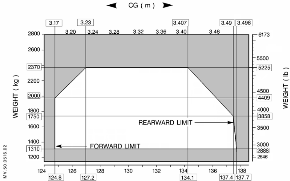
CG (in) Longitudinal: AS350 B3 ARRIEL 2D:
