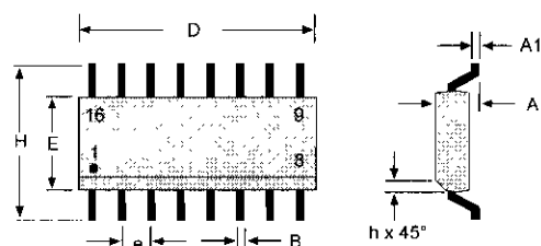
HMC1022—16-Pin SOIC
