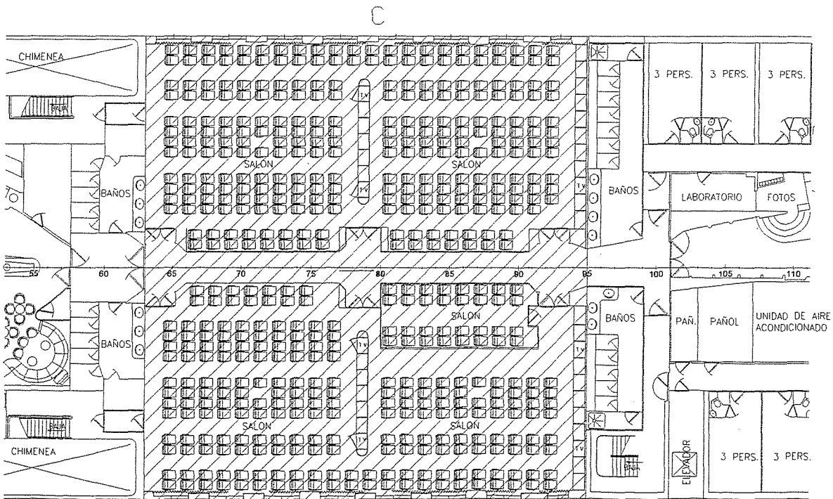
CUBIERTA 6
