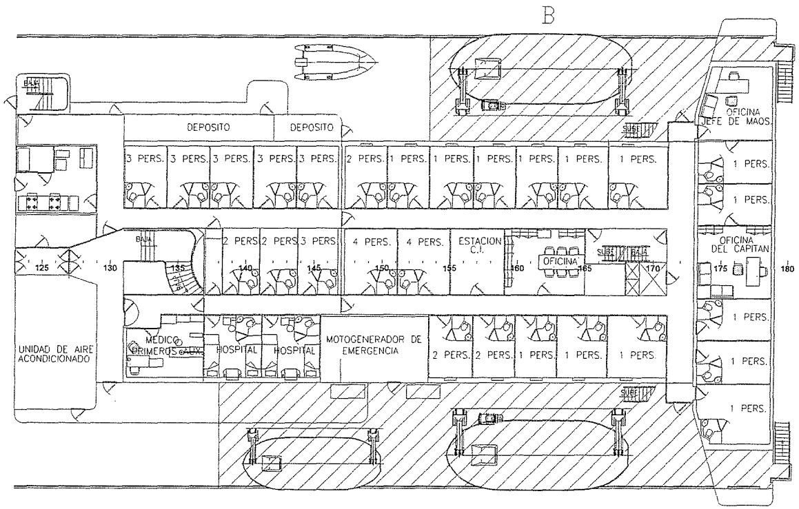
CUBIERTA 7
